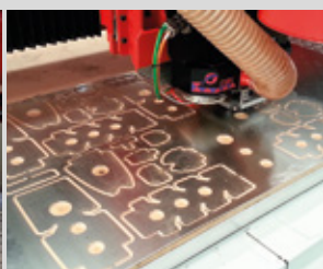
Nesting lamiere a pacco in alluminio
